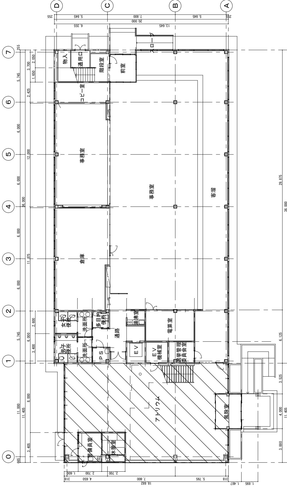
1 階平面図
