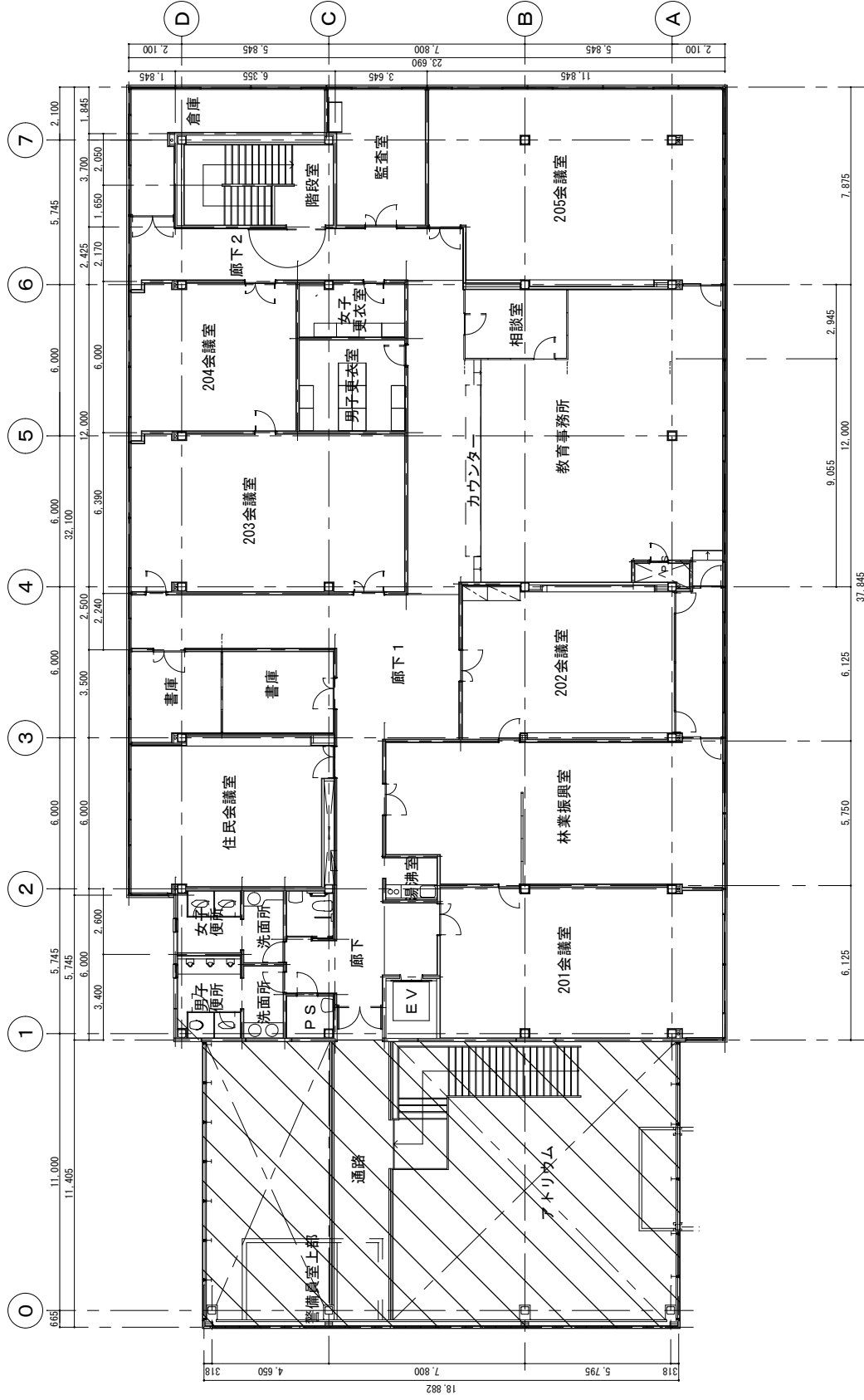
2階平面図
