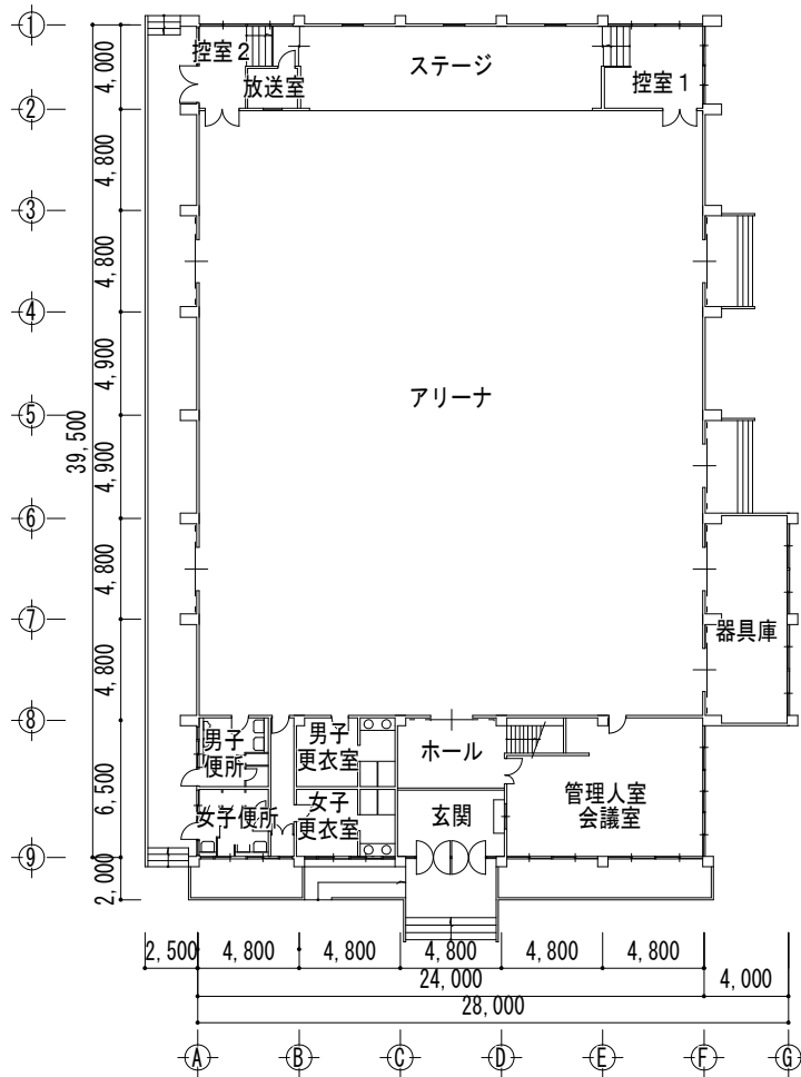
1 階平面図
