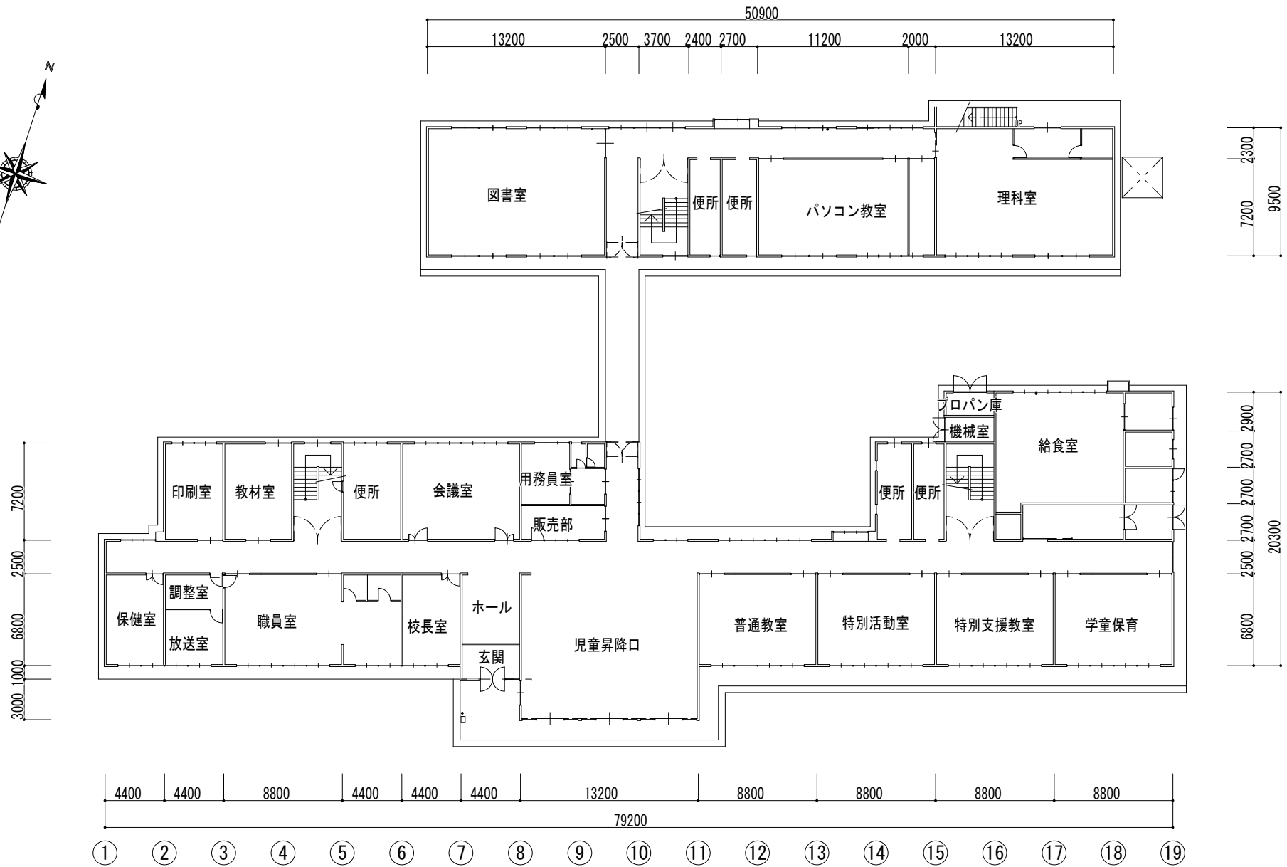
1階平面図
