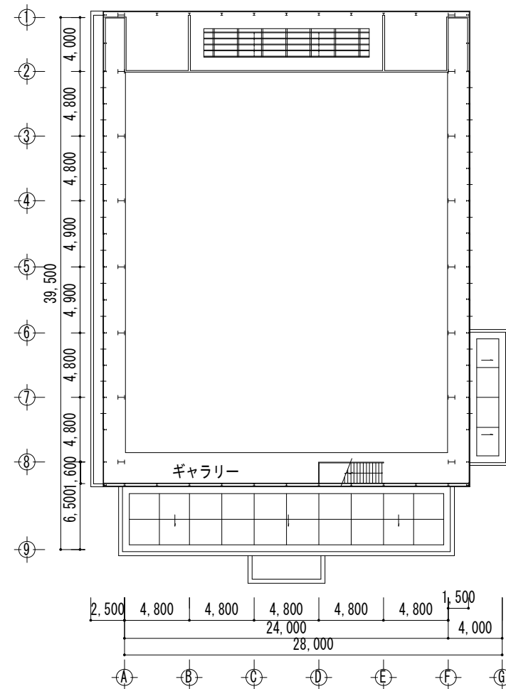
2 階平面図
