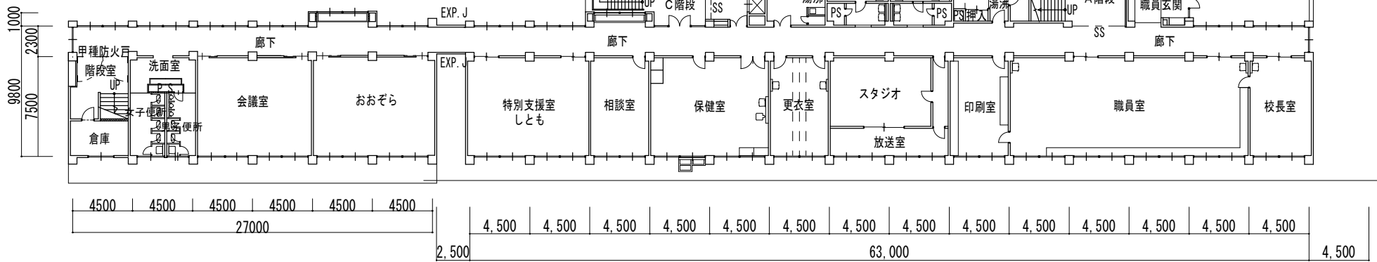
1階平面図
