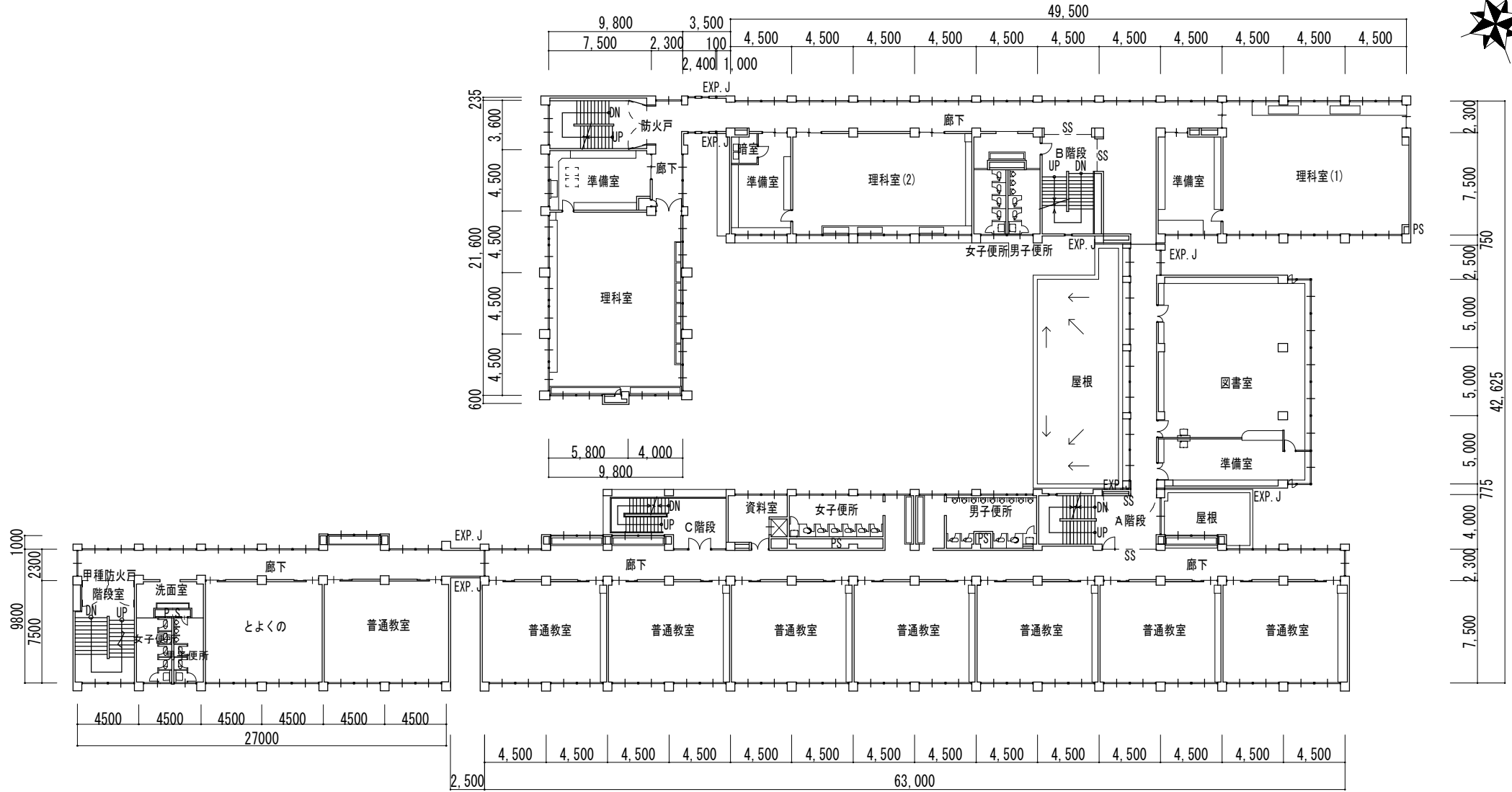
2階平面図
