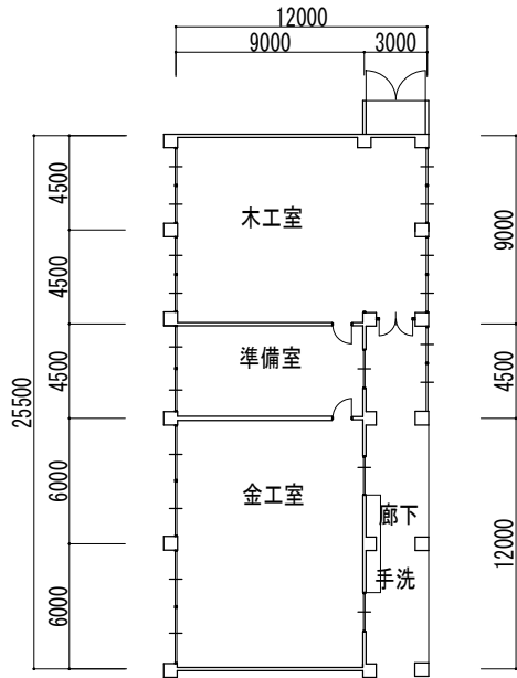
技術棟平面図
