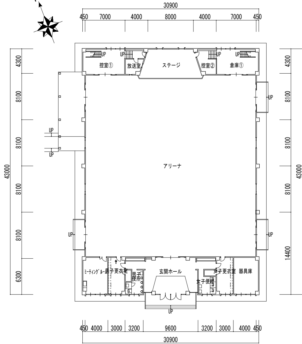
1階平面図
