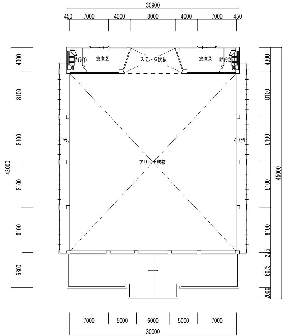
2階平面図
