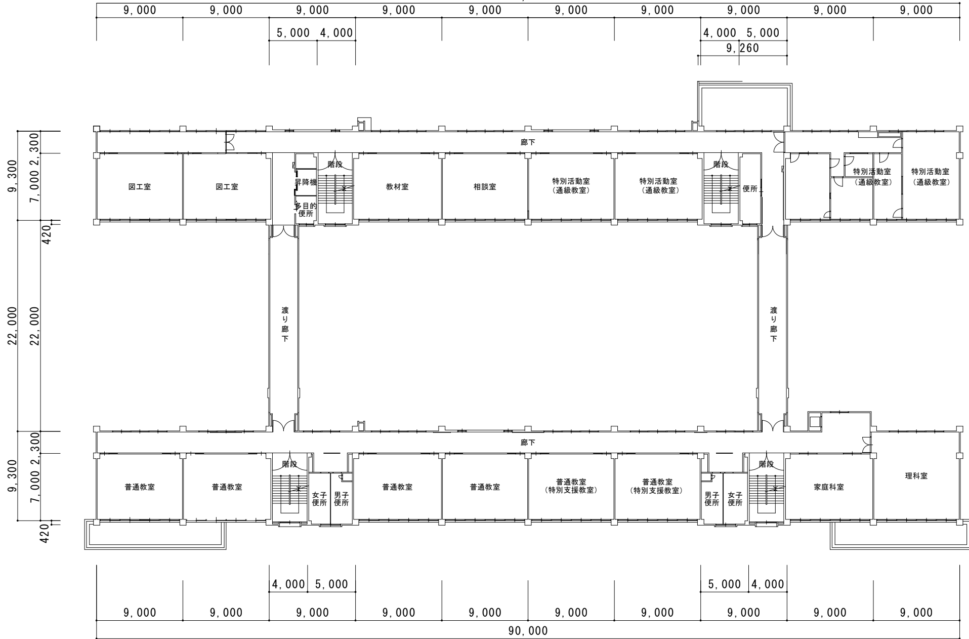
2階平面図
