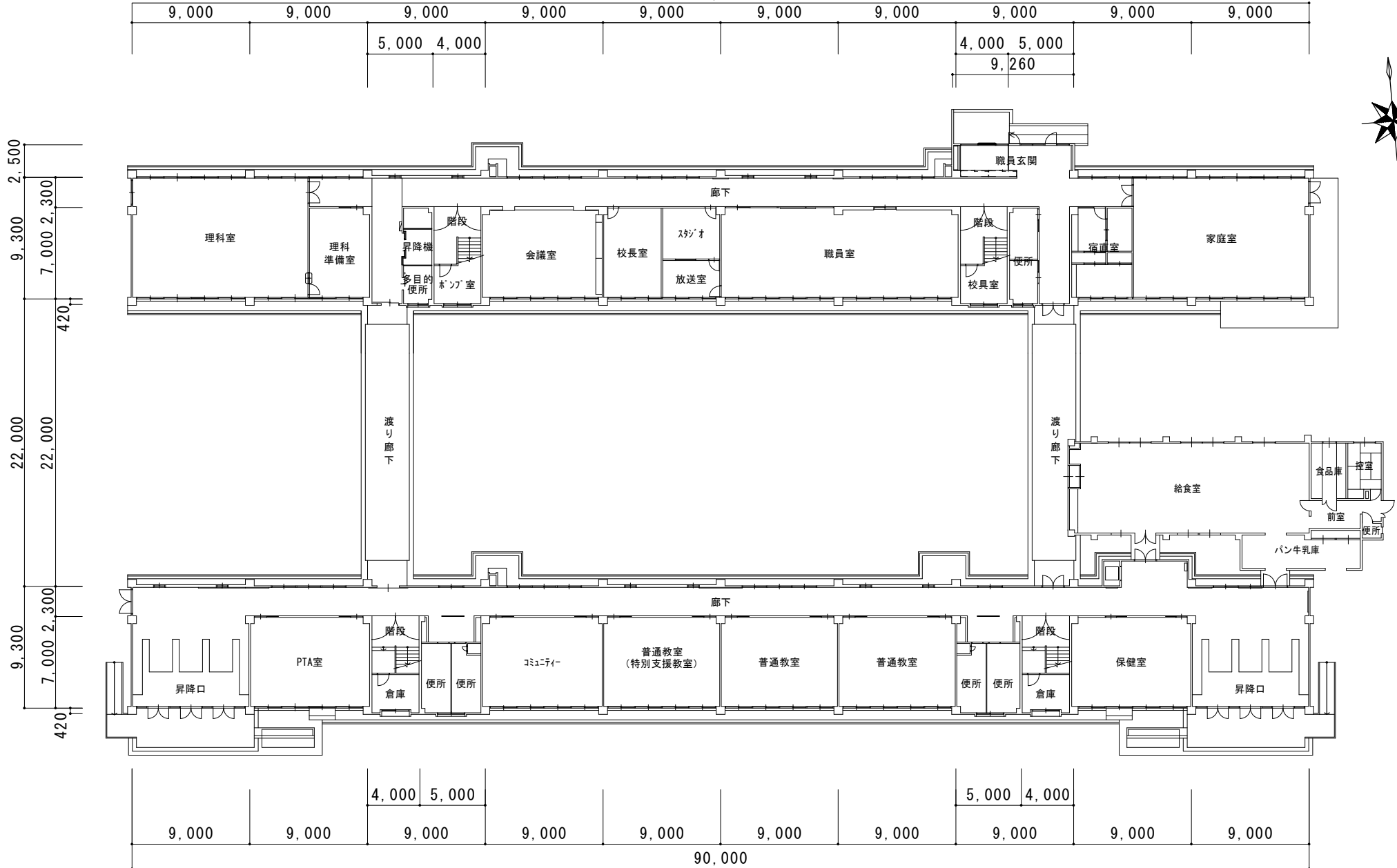
1階平面図
