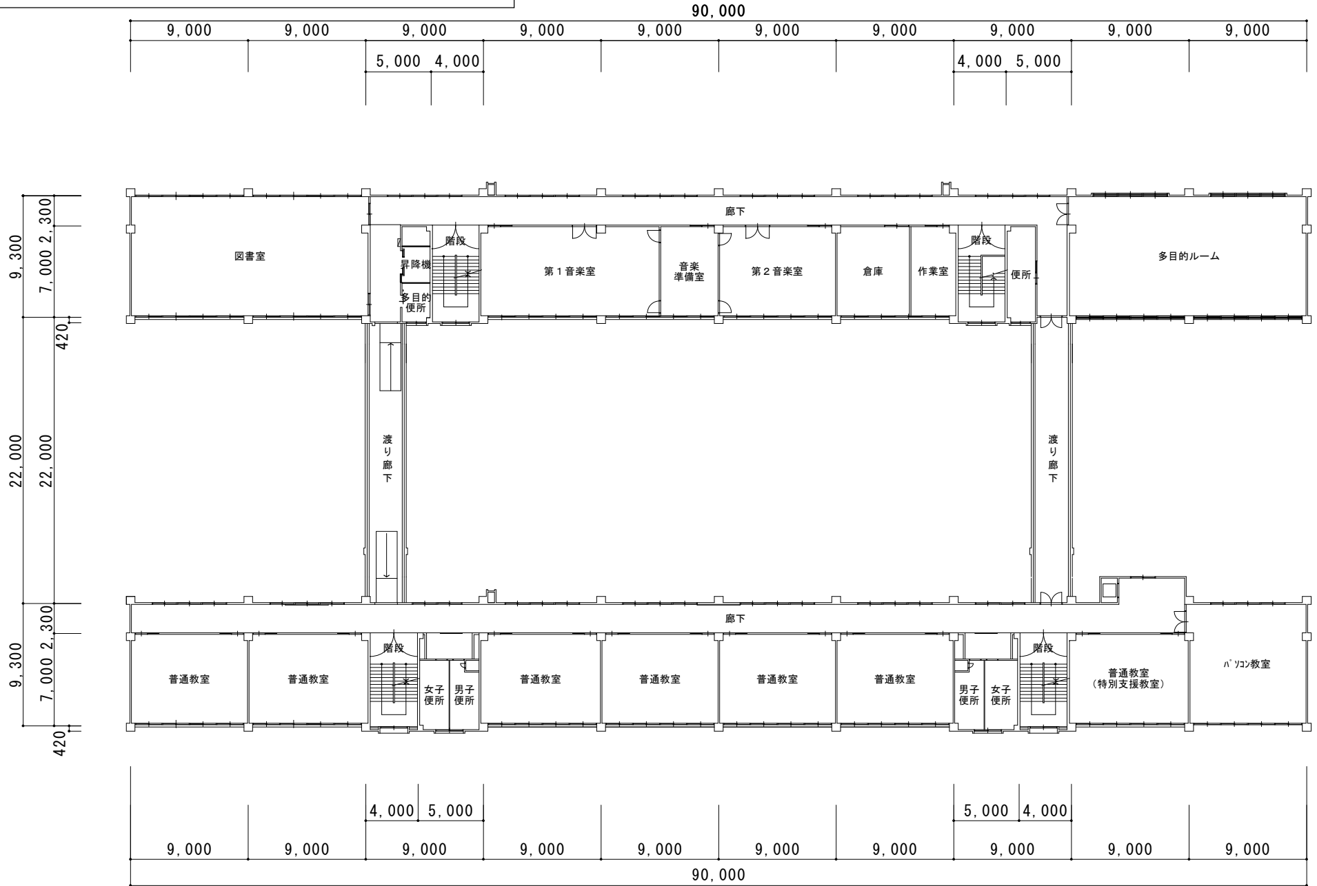
3階平面図
