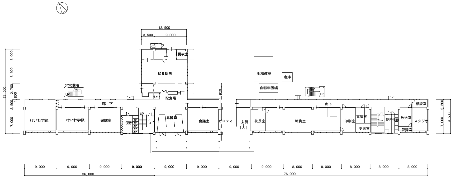
1 階平面図
