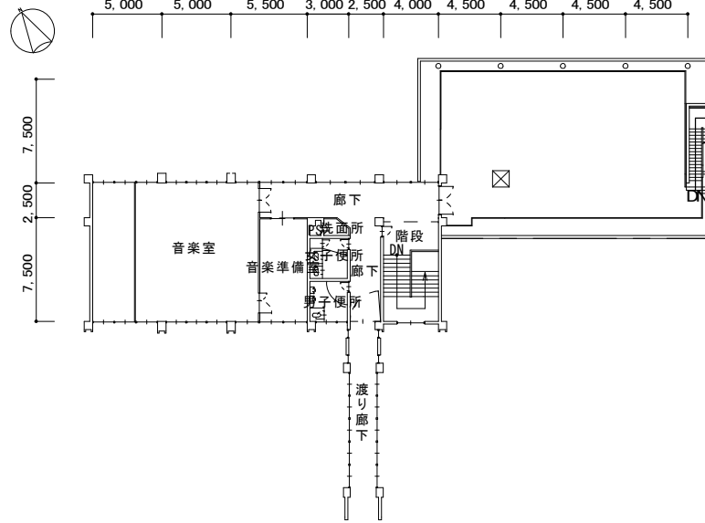
3階平面図
