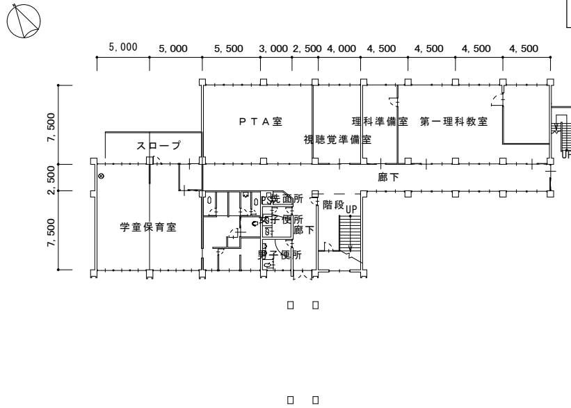
3階平面図
