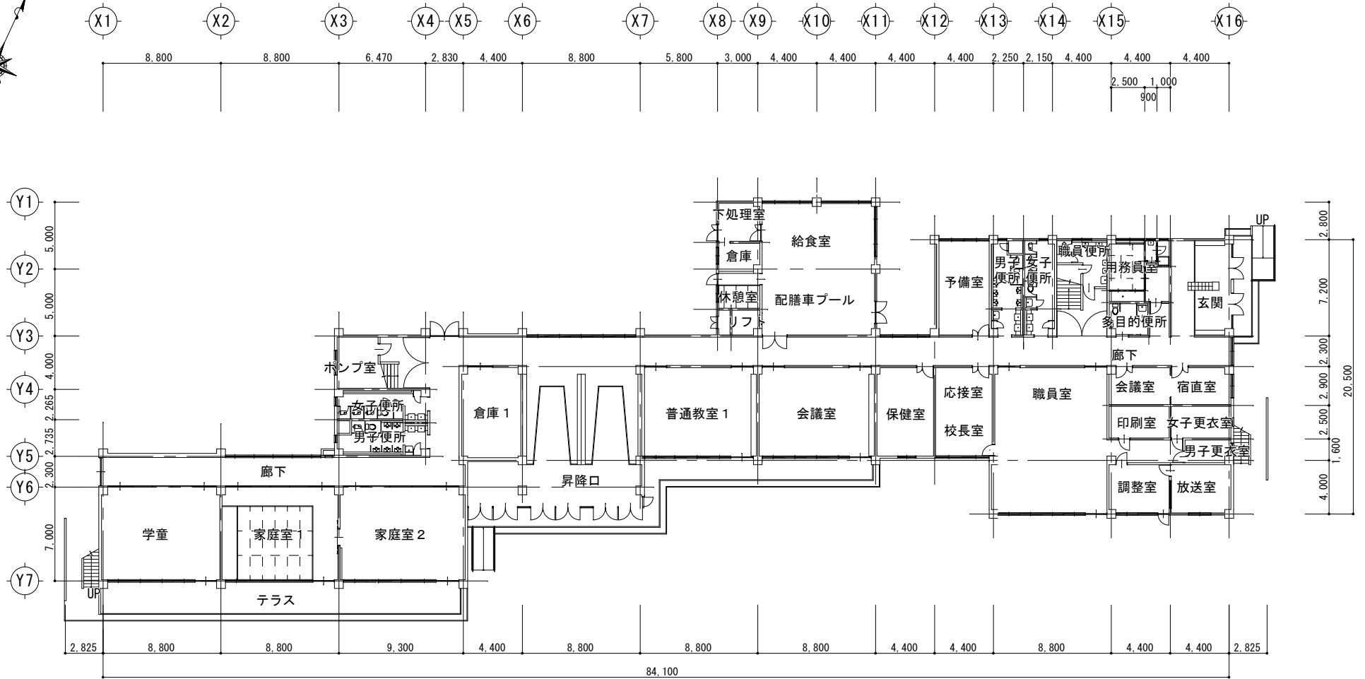
1階平面図
