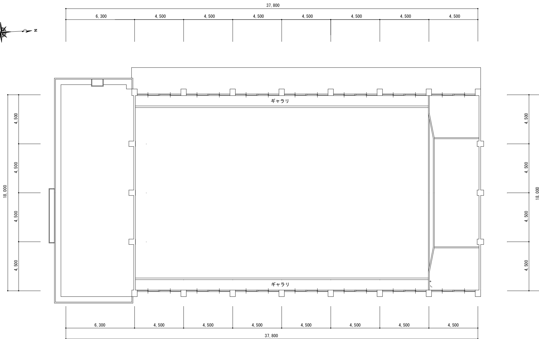
2階平面図
