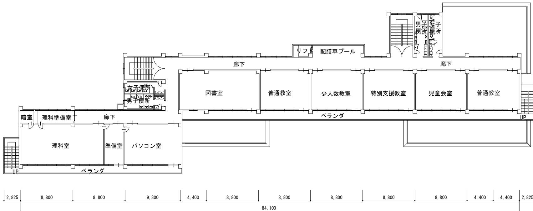
2階平面図
