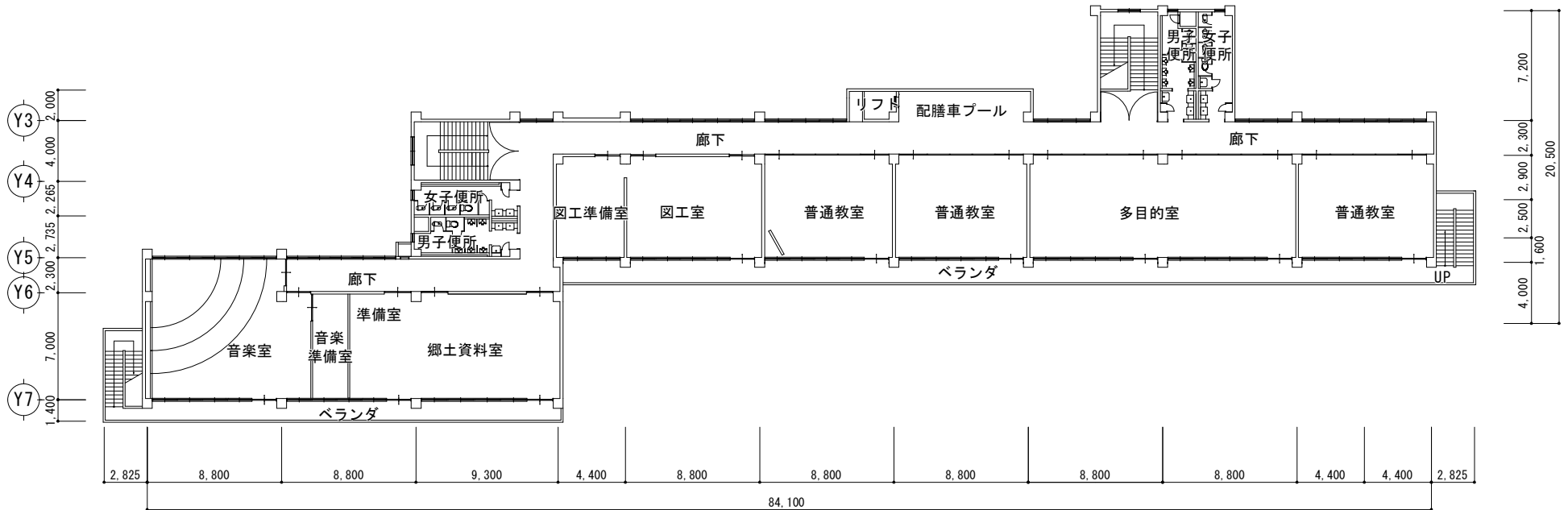
3階平面図
