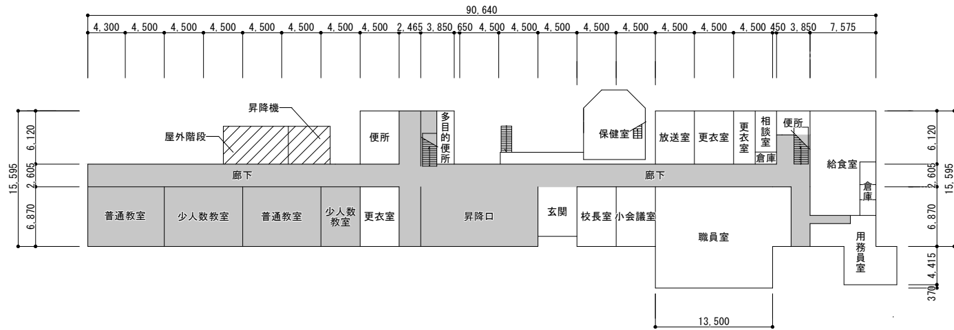
1階平面図
