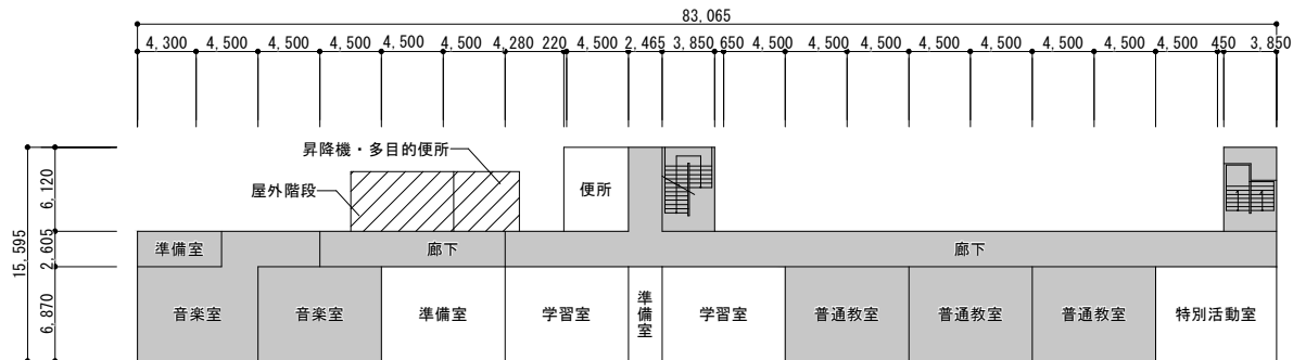
3階平面图
