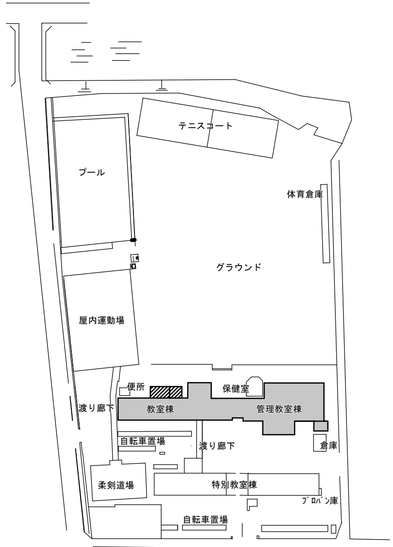
配置図
