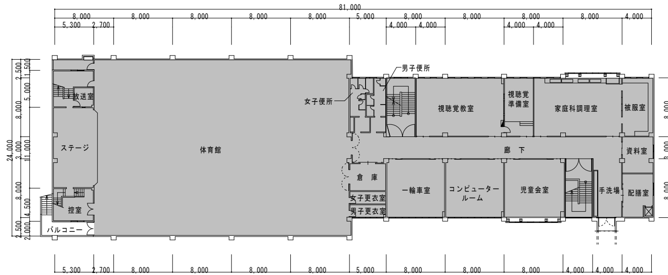
3階平面図
