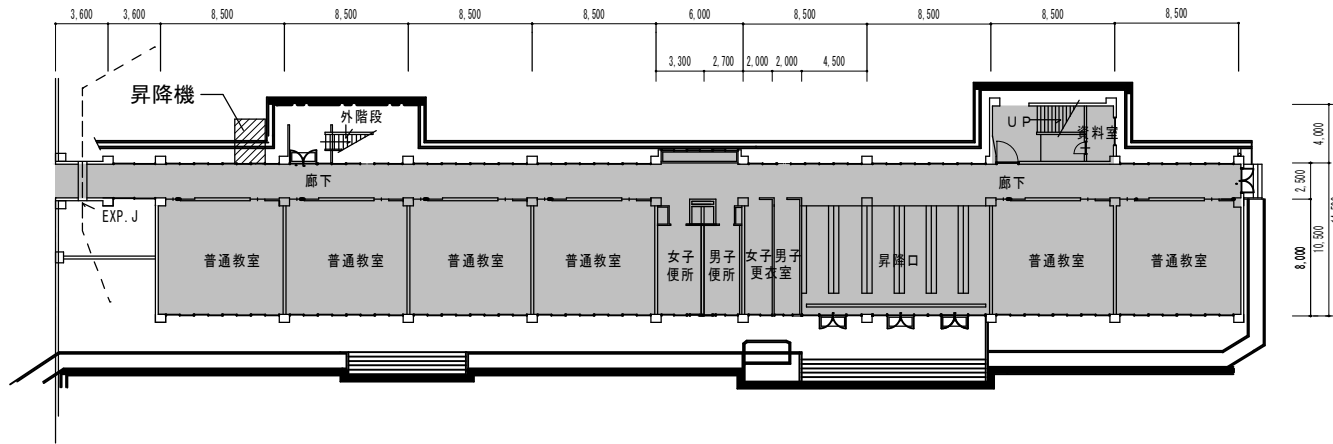
1階平面図
