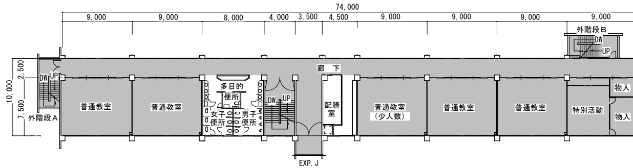
3階平面図
