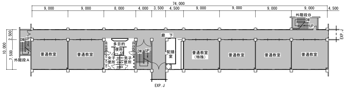
2階平面図
