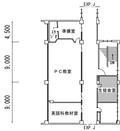
4階平面図
