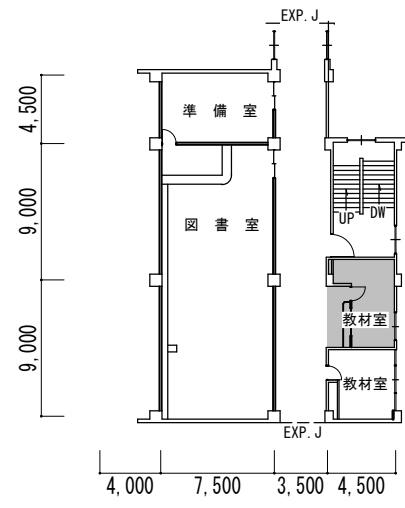
3階平面図
