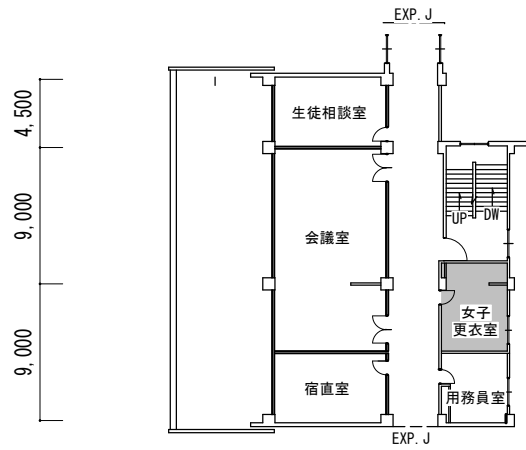
2階平面図
