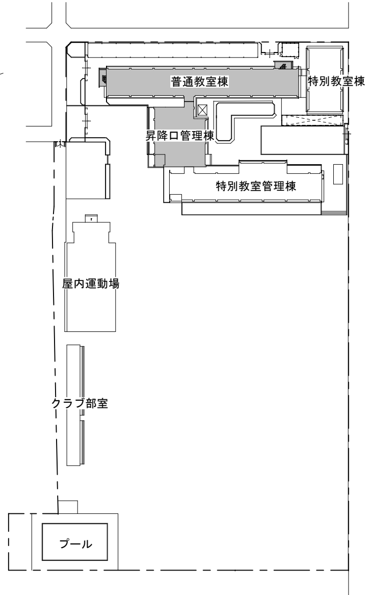
配置図
