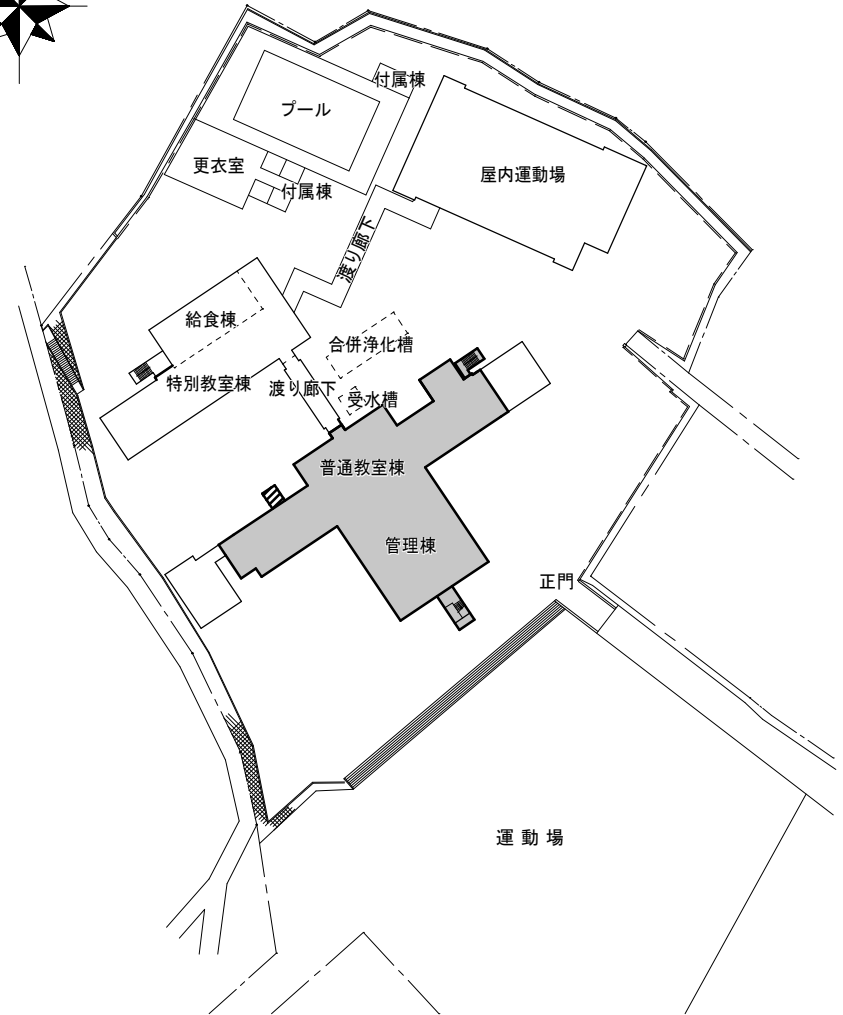
配置図
