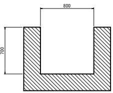
現場打ち水路 (800 × 700) S=1:20
