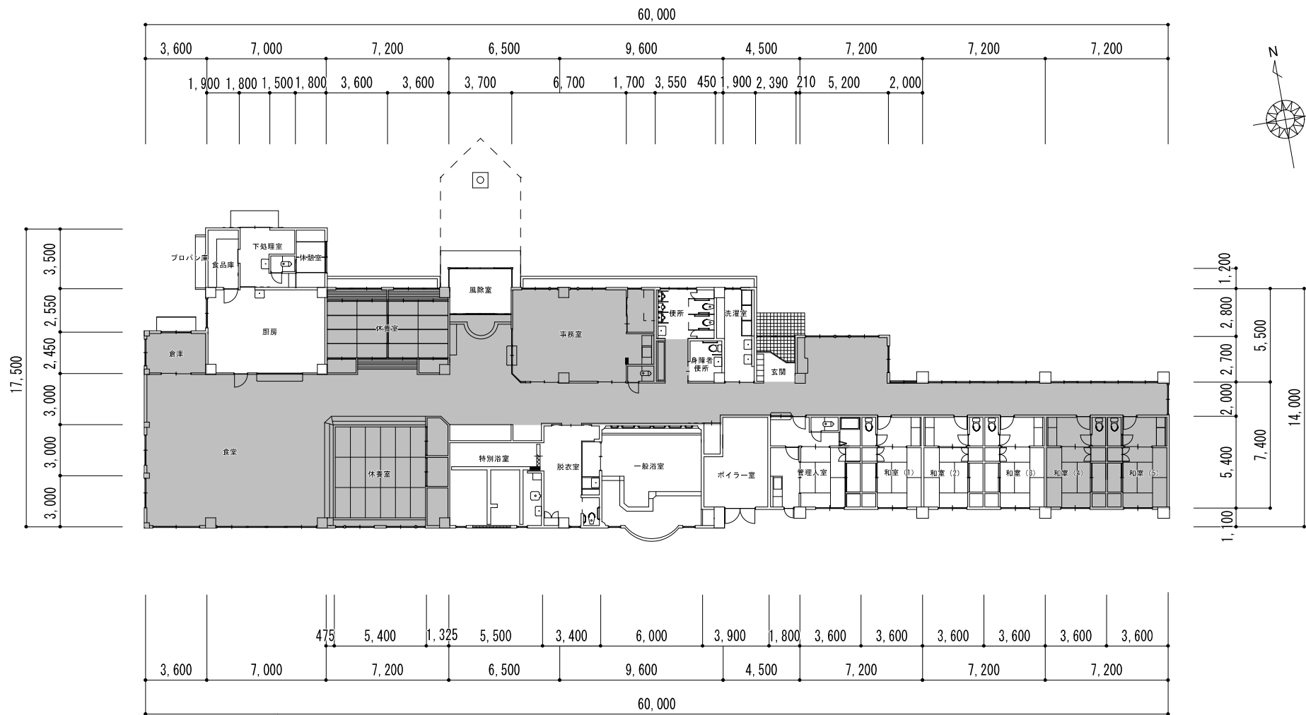
平面図
