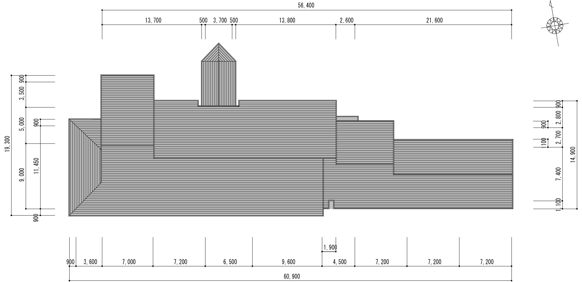
屋根伏図
