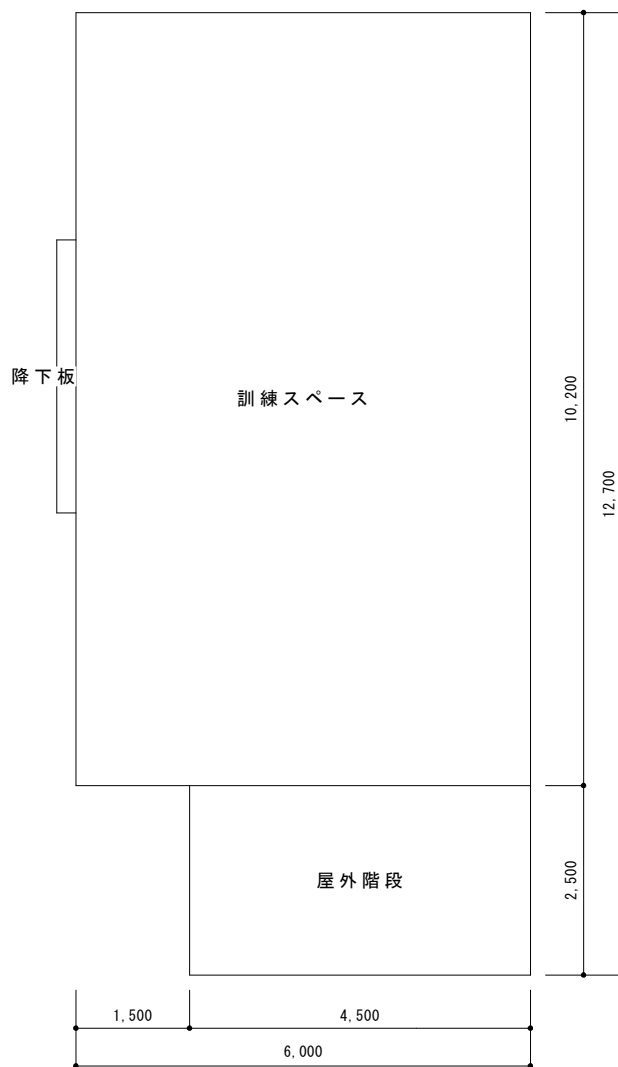
2階平面図 (参考)
