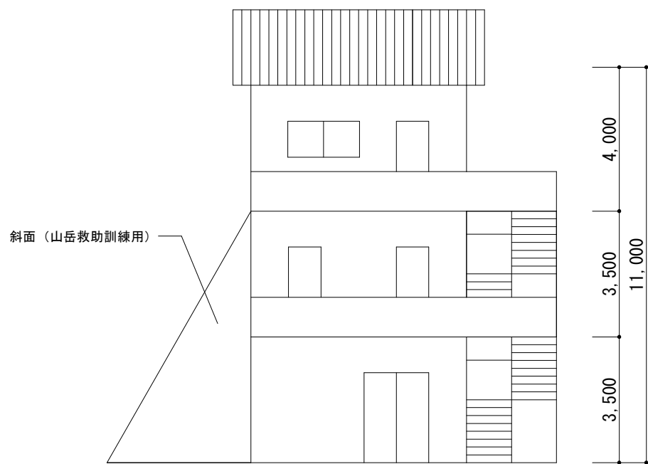
主訓練塔 西立面図 (参考)
