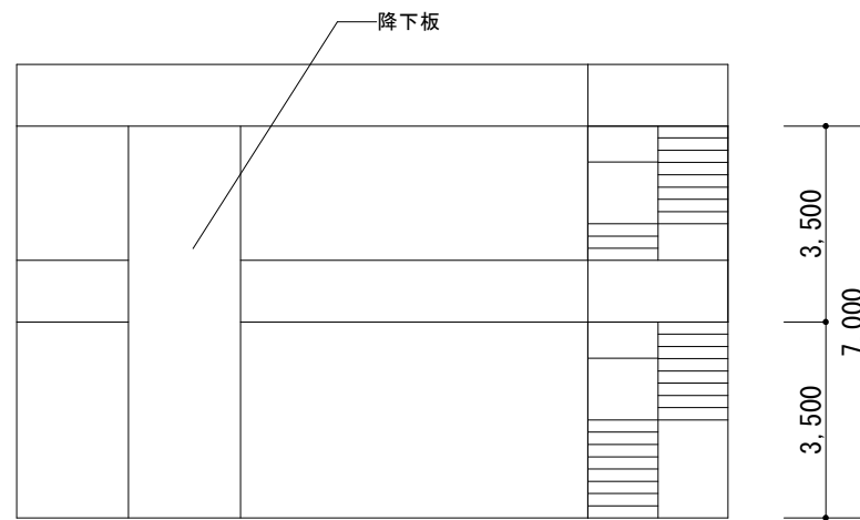
補助訓練塔 西立面図 (参考)
