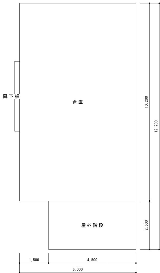
1階平面図 (参考)
