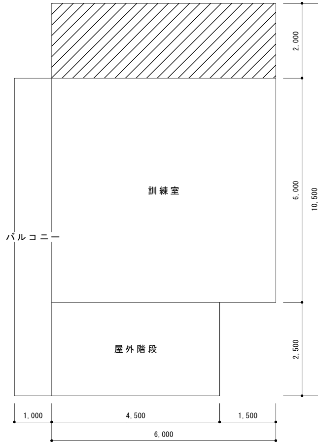
2階平面図 (参考)
