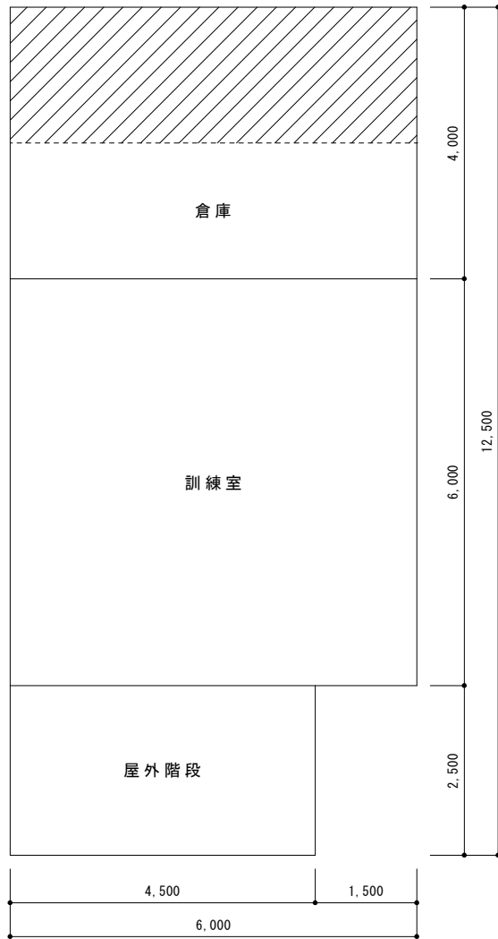
1階平面図 (参考)
