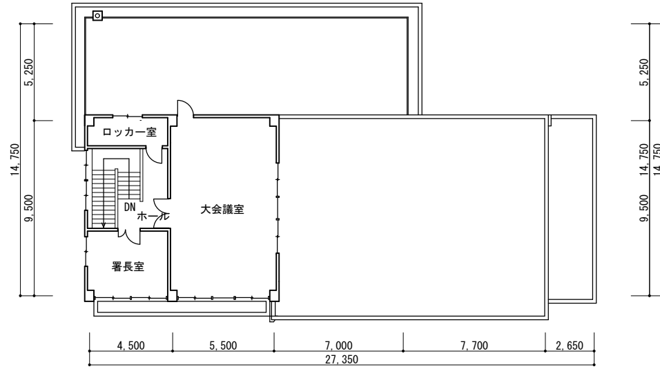
2階平面図
