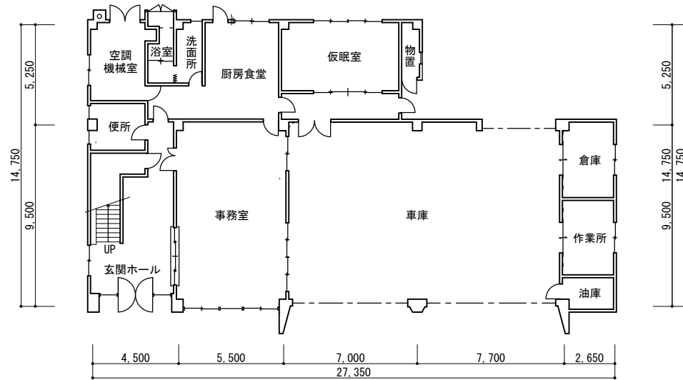
1階平面図
