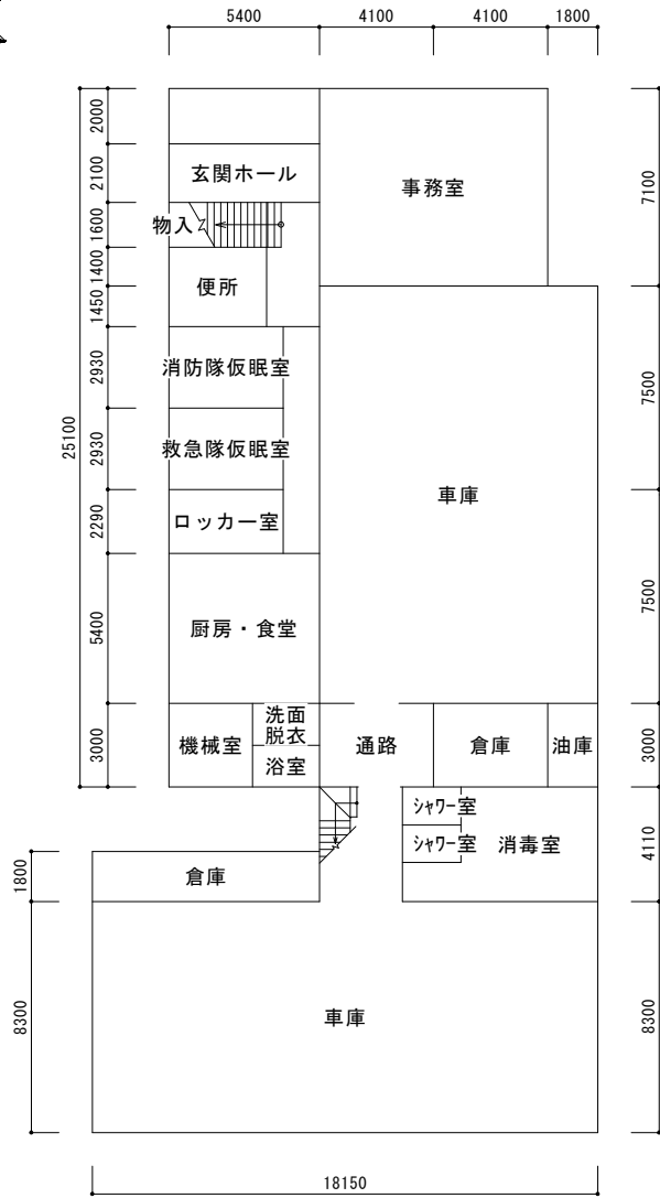
1階平面図
