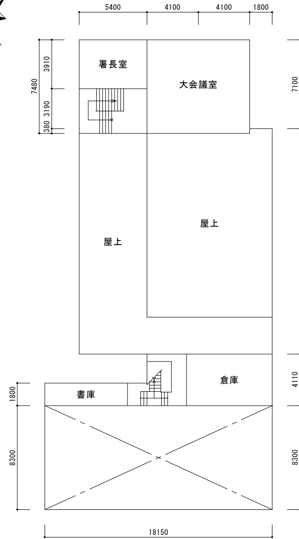
2階平面図
