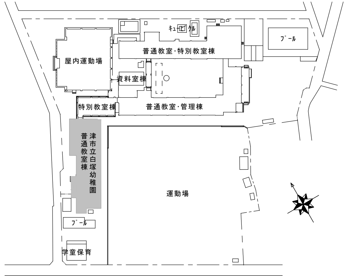
配置図
