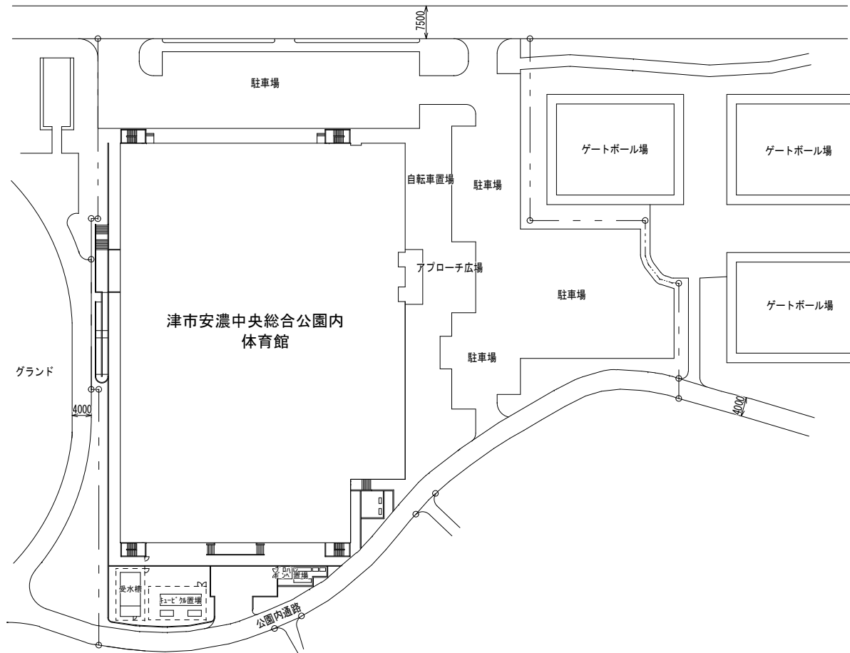
配置図
