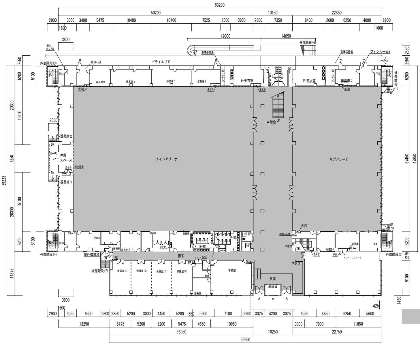
1階 平面図
