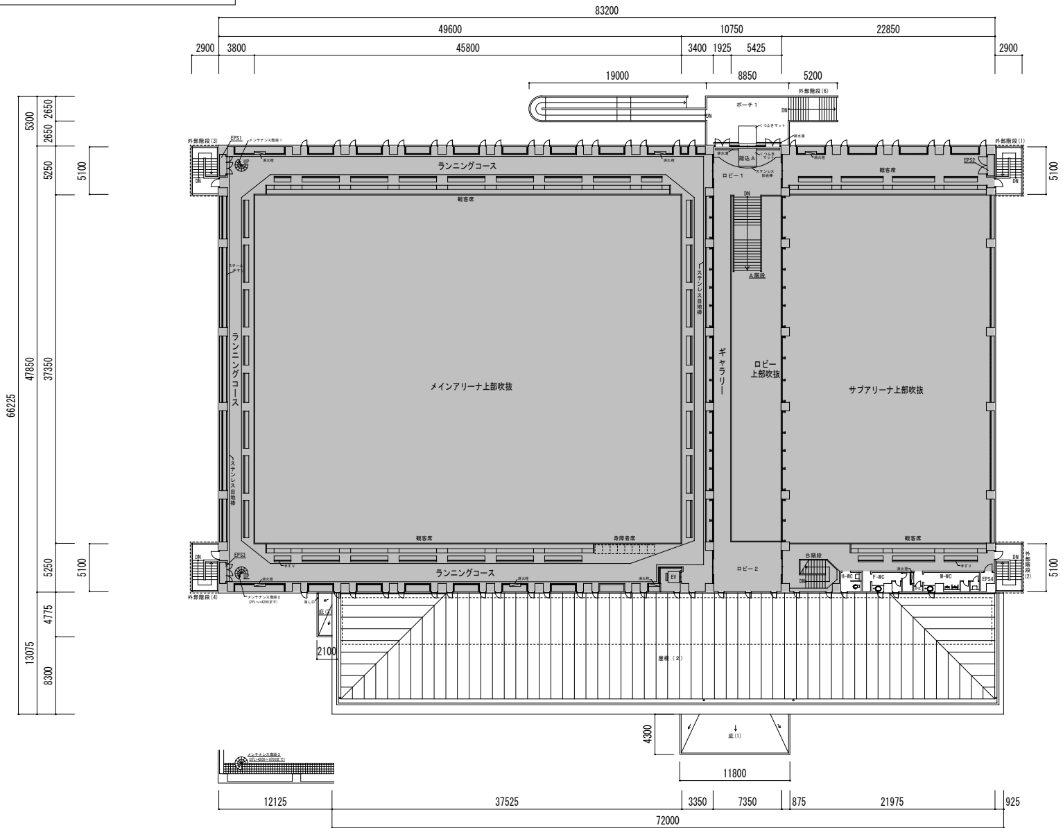
2階 平面図
