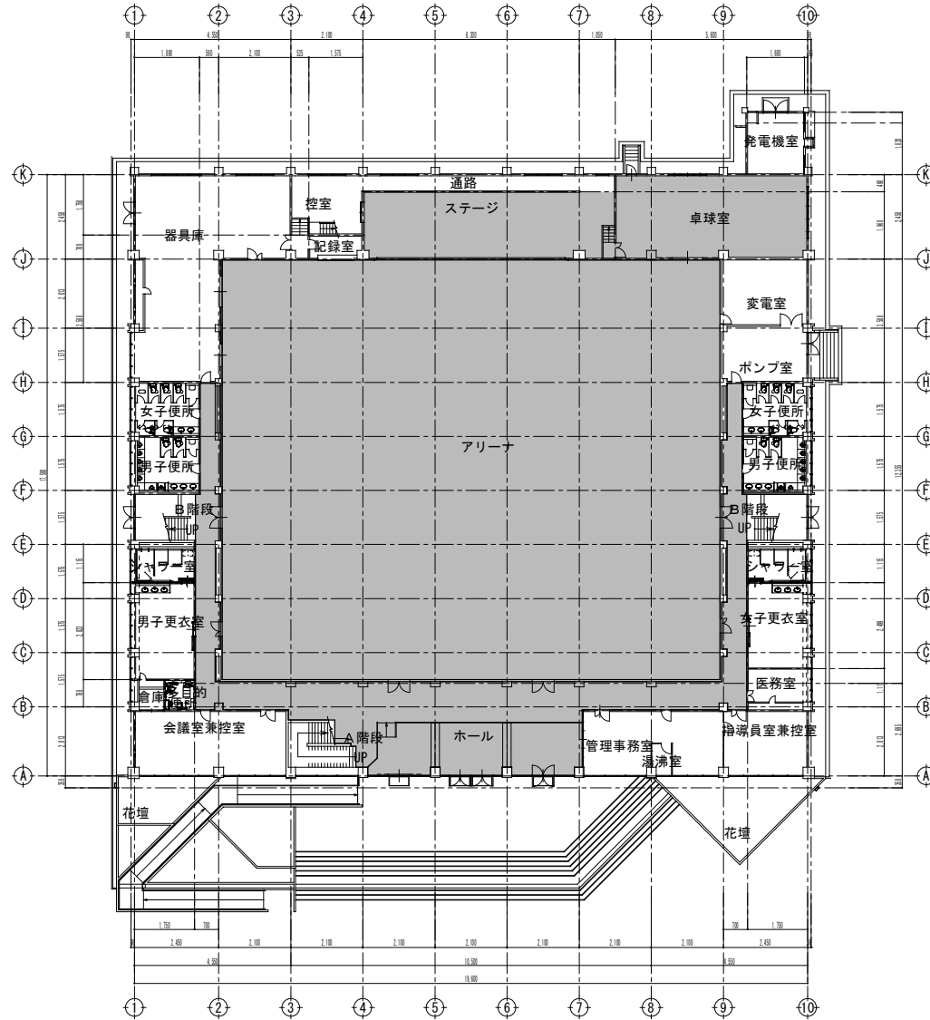
1階 平面図
