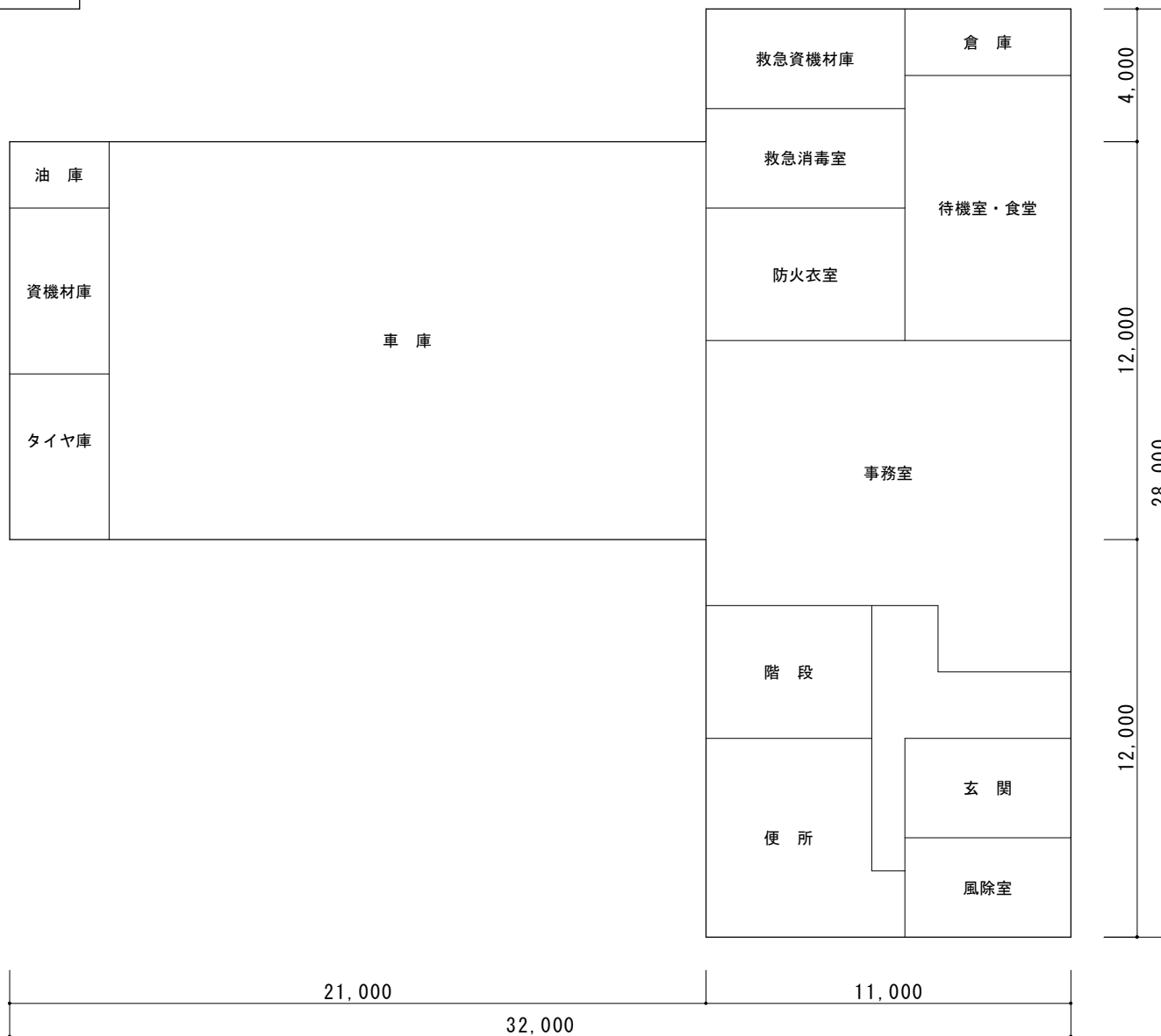
1階平面図(参考)
