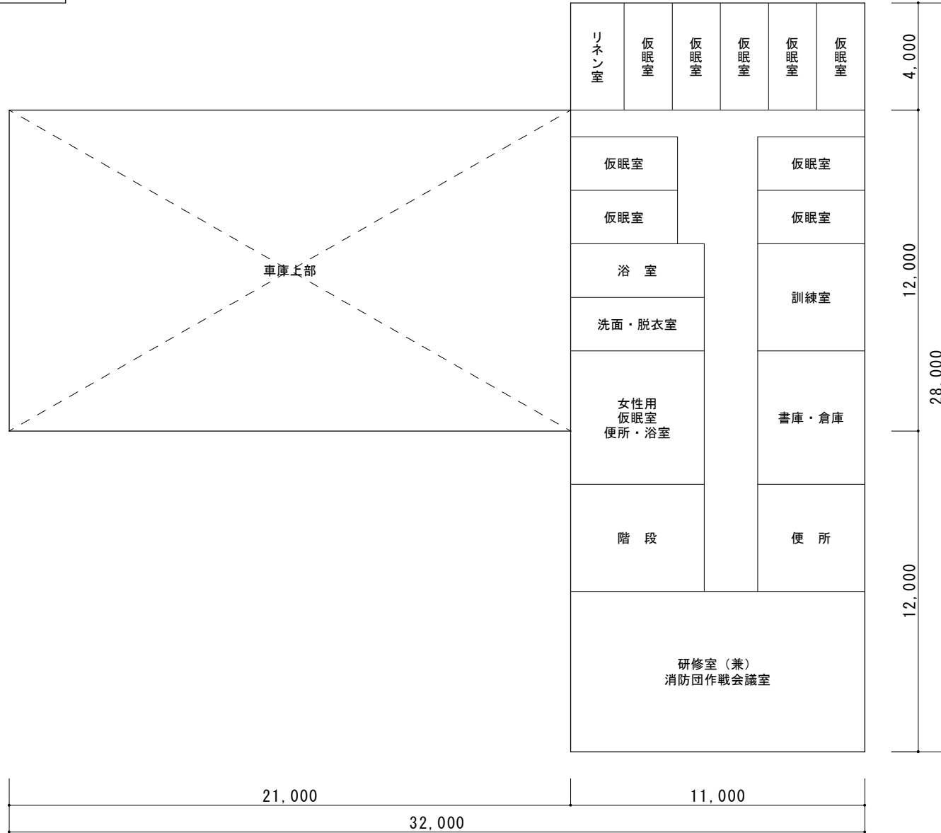
2階平面図(参考)
