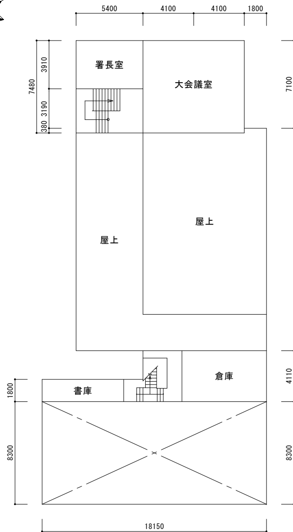
2階平面図
