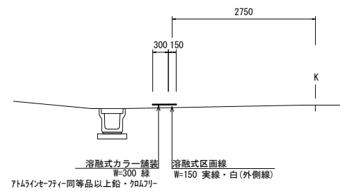
A-A' 断面
