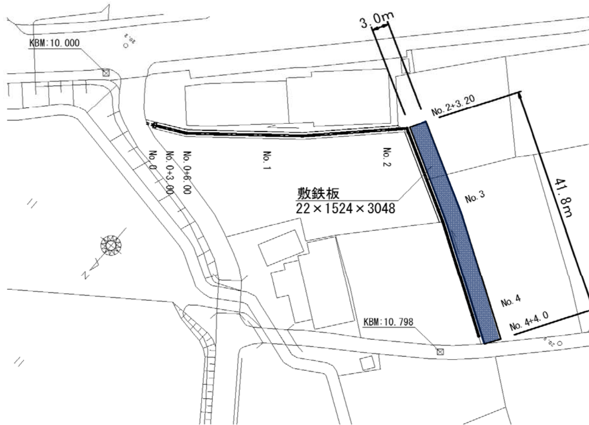
仮設平面図
