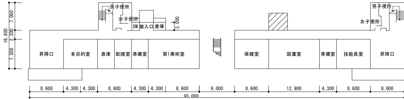
1階平面図
