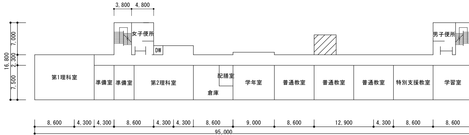
3階平面図
