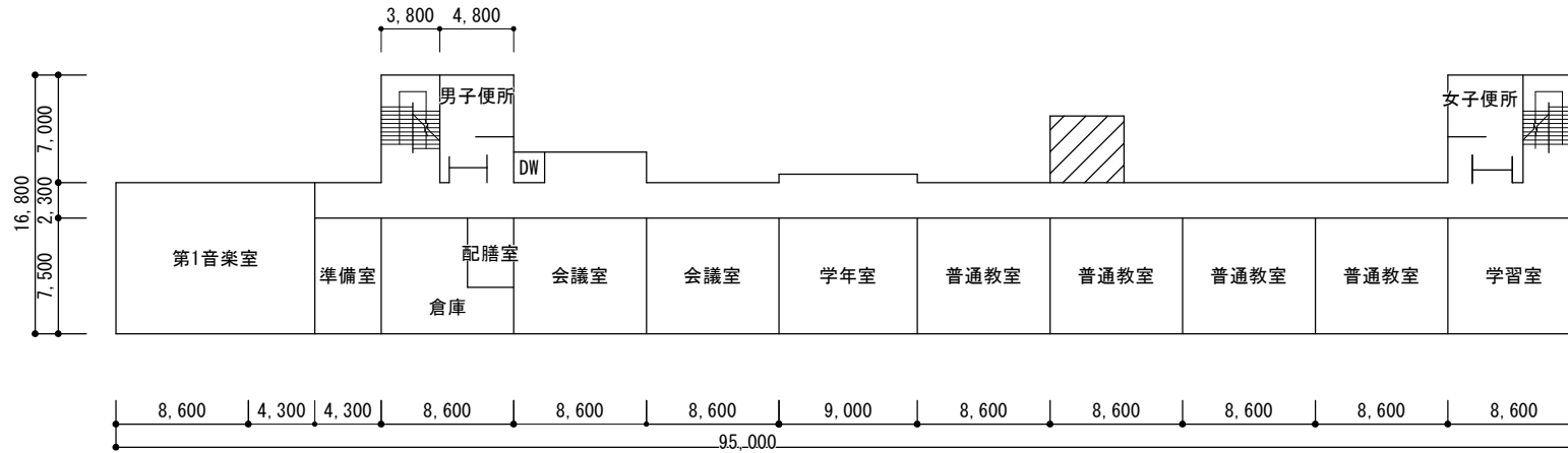
4階平面図
