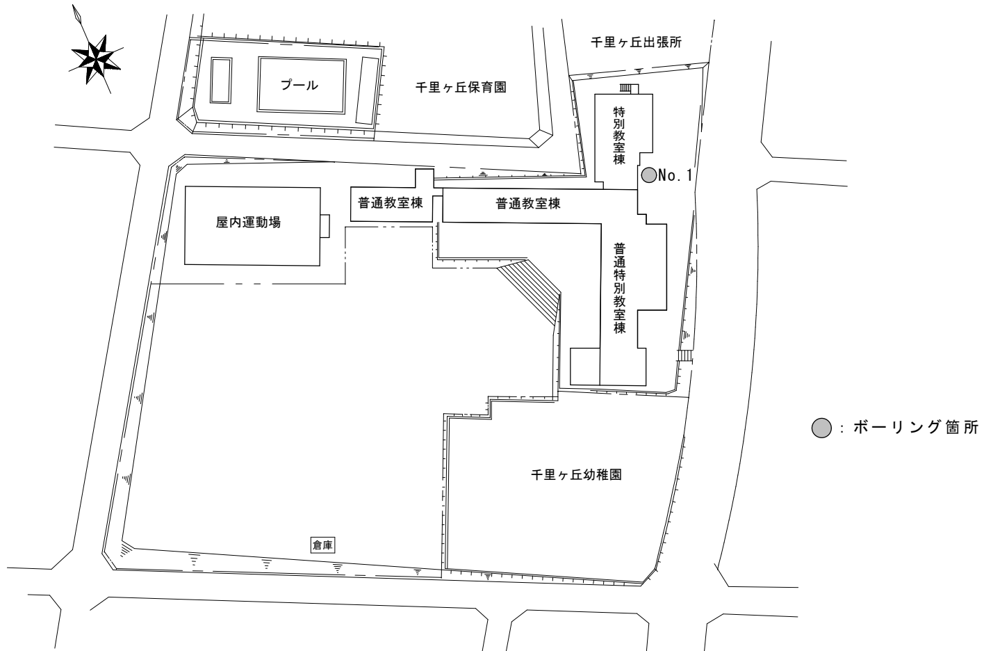
配置図
