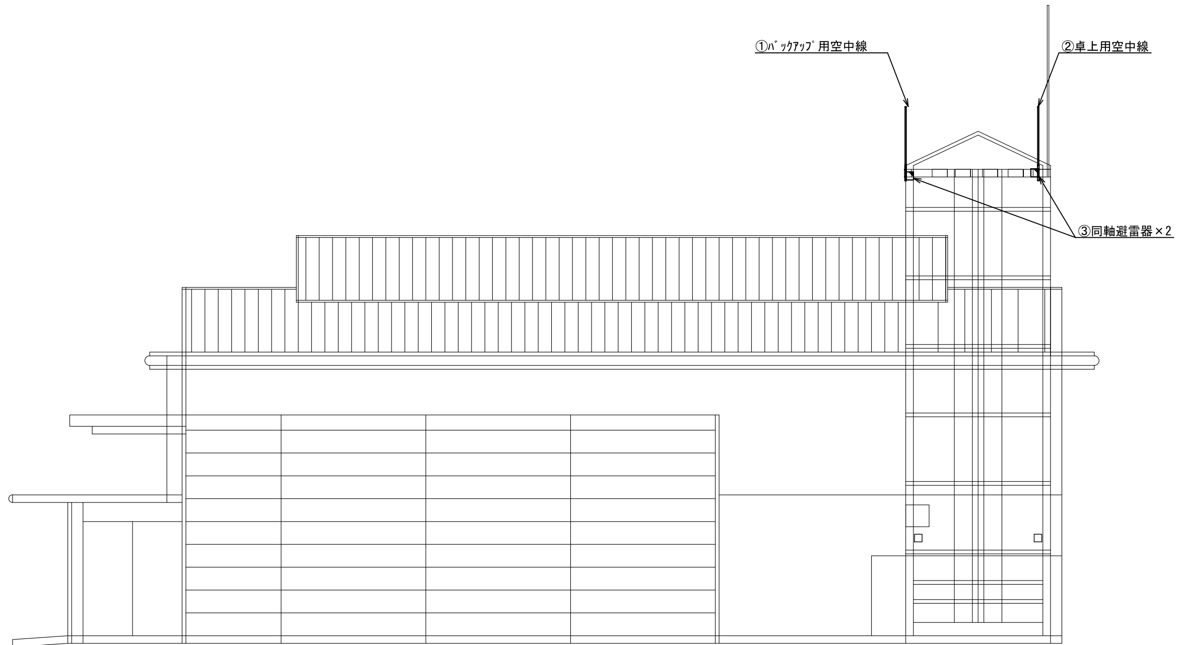
西立面図
