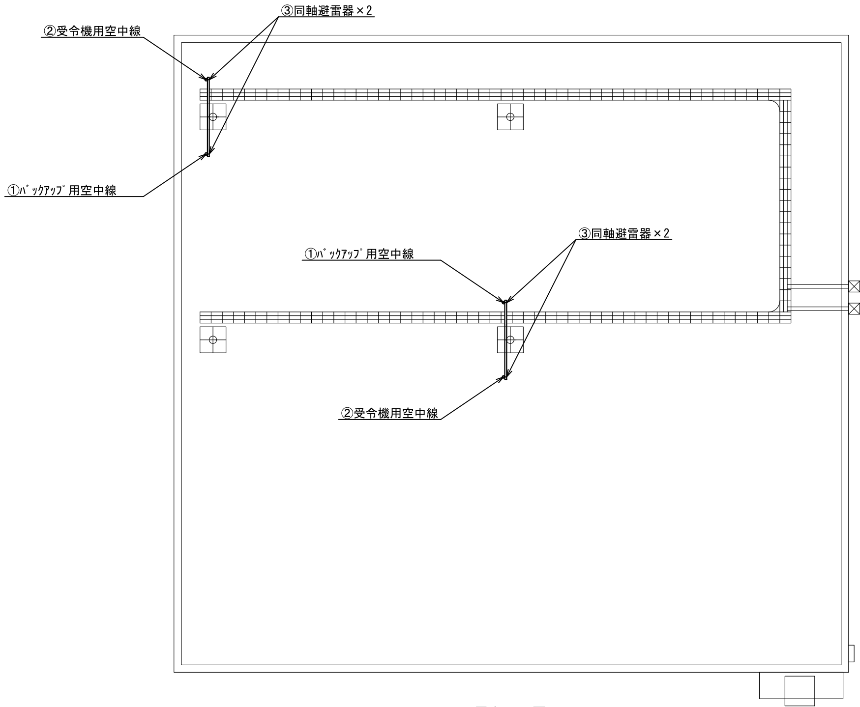
屋上平面図
