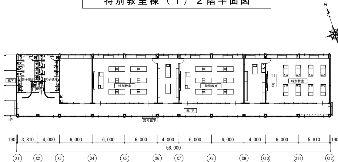
特別教室棟（２）１階平面図
