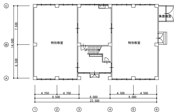
特別教室棟（１）１階平面図
