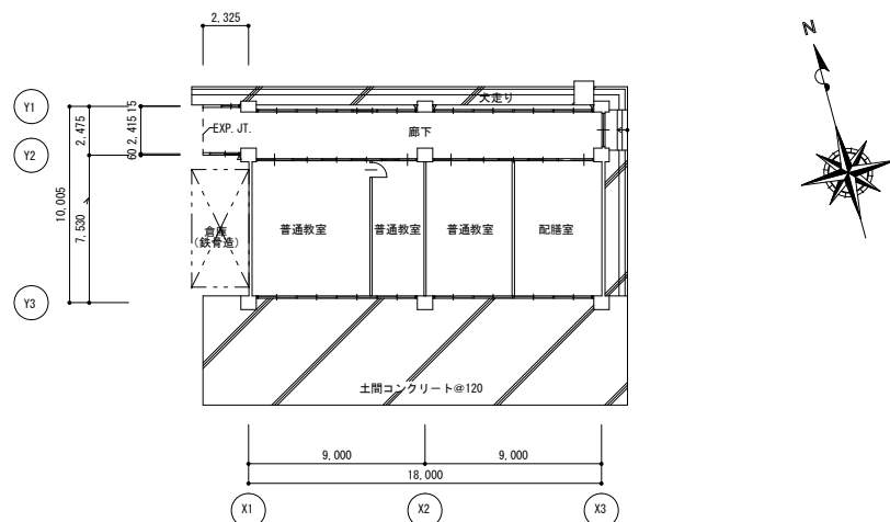
1 階平面図
