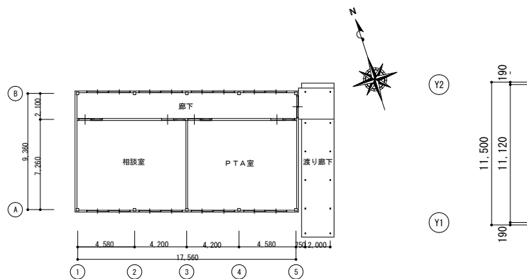
特別教室棟（１）１階平面図
