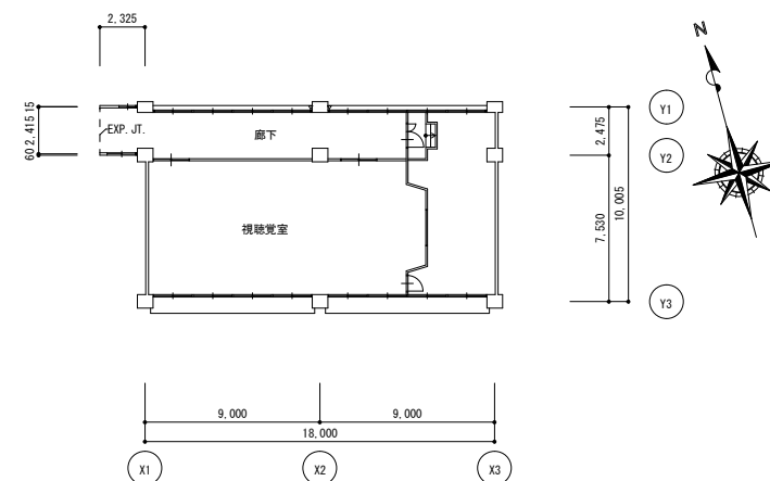
4 階平面図
