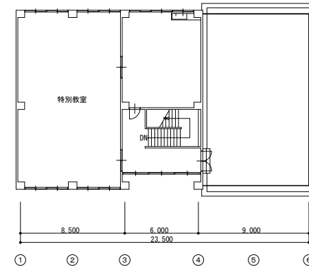
特別教室棟（１）２階平面図
