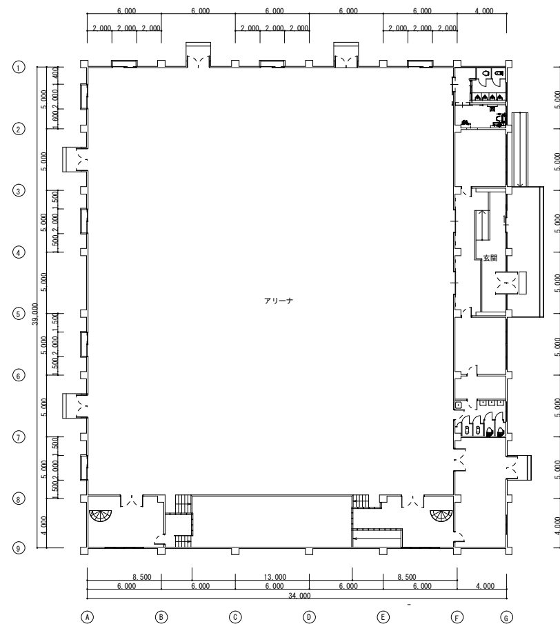
1 階平面図
