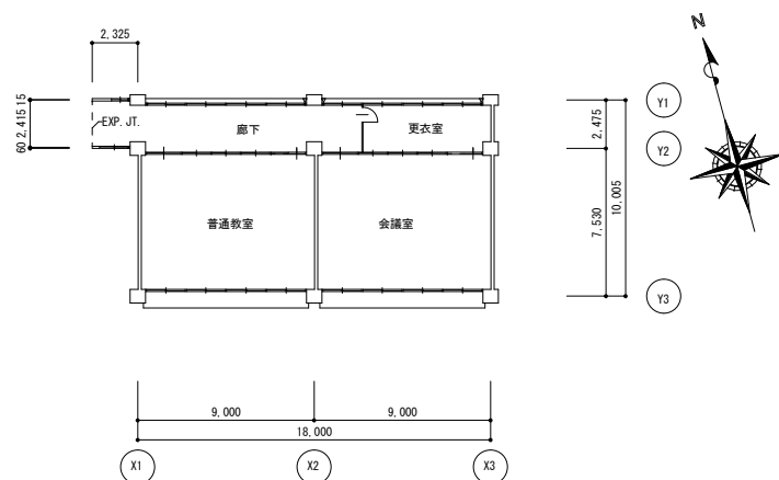
2 階平面図
