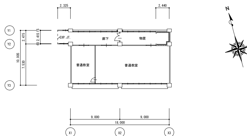
3 階平面図
