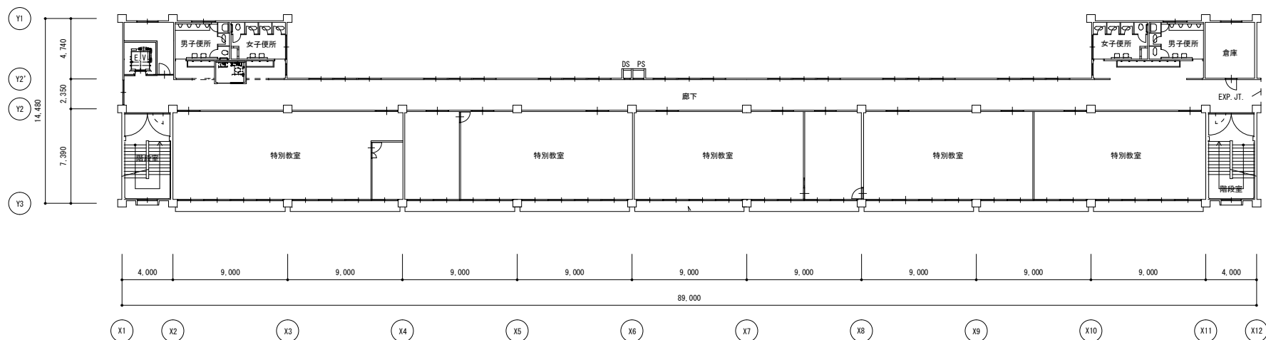
4 階平面図
